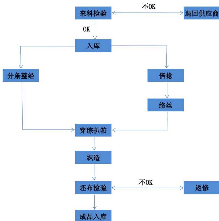
生产流程图
